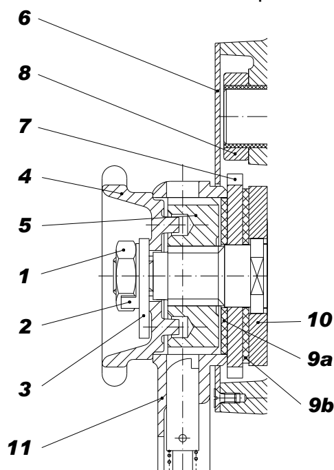
Рис. 11.3. Монтаж тормоза
