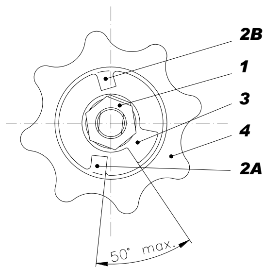
Рис. 11.4. Регулировка тормоза
